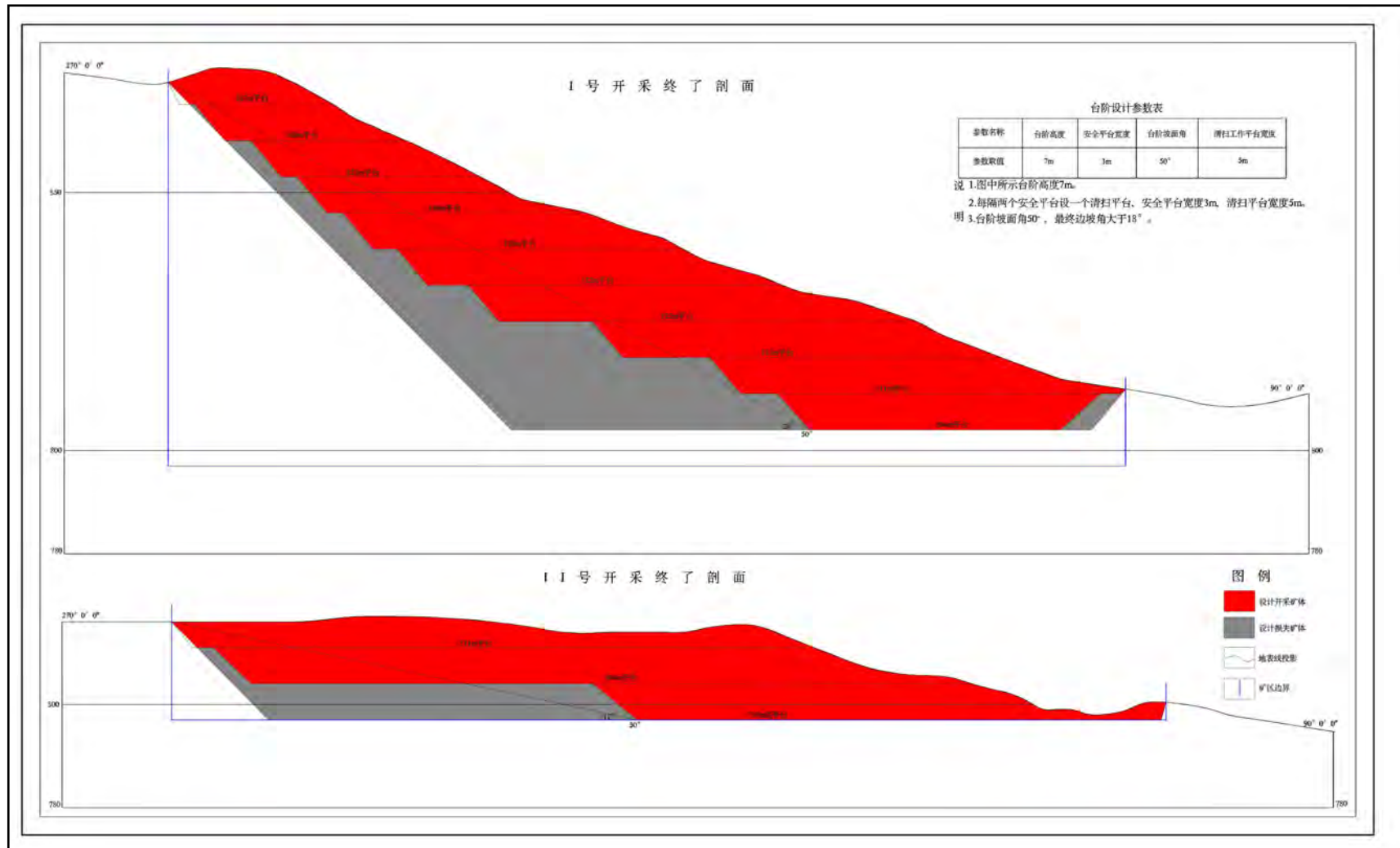
图 1-5 开采剖面图 (1:1000)
