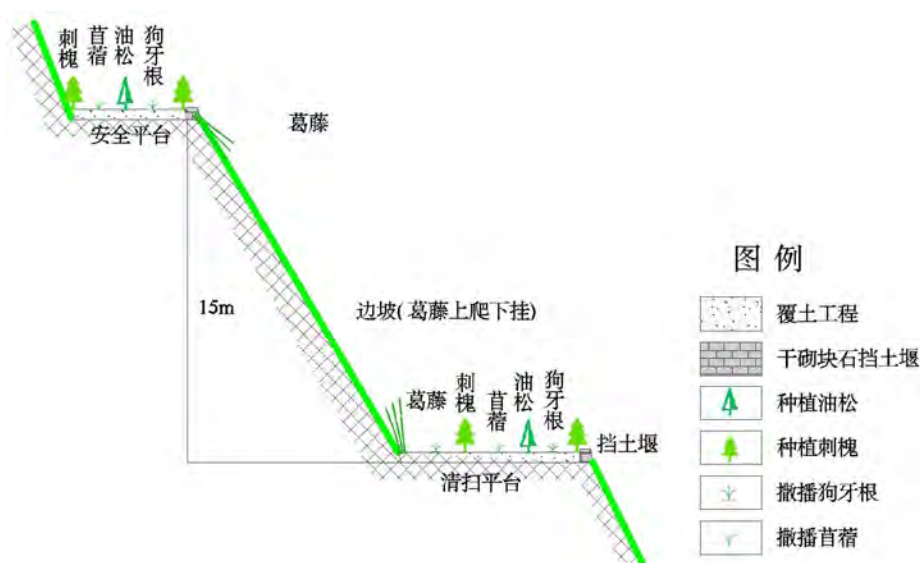
图 5-5 采场平台林地治理剖面图
