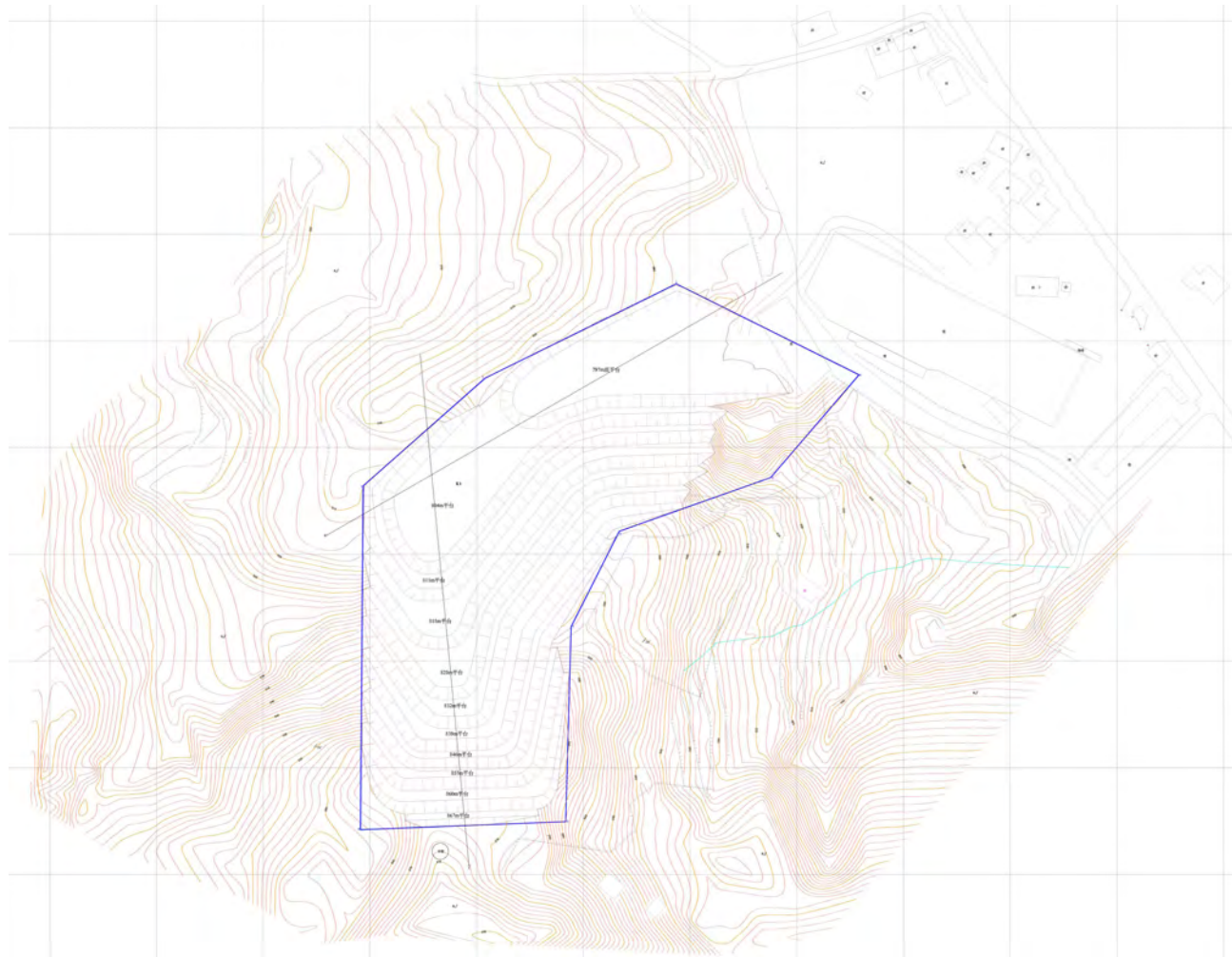
图 1-4 最终开采终了平面图 (1: 500)
