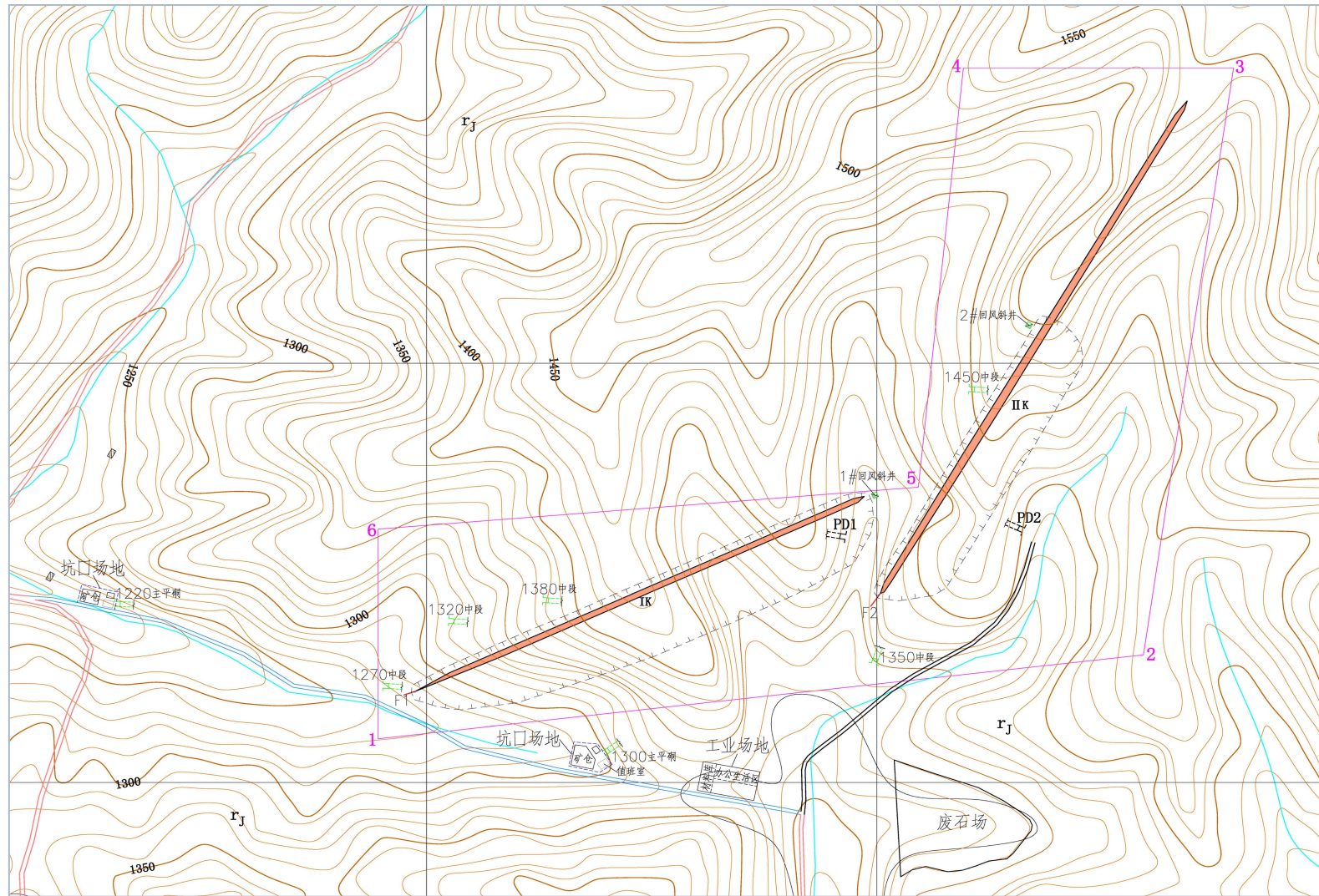
图 1-4 矿山总平面布置图
