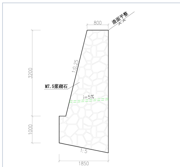
图 5-1 拦渣挡墙断面设计图
