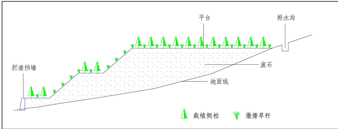
图 5-4 废石场复垦植树典型设计图
