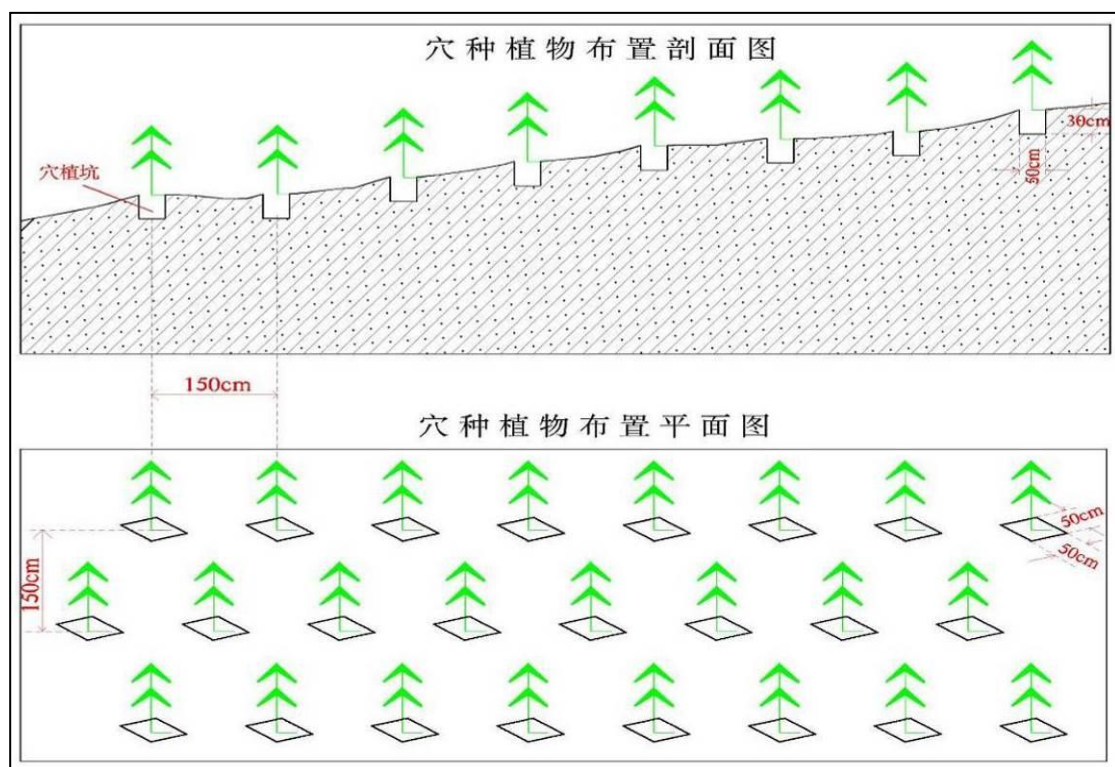
图 5-5 栽植乔木典型设计图
