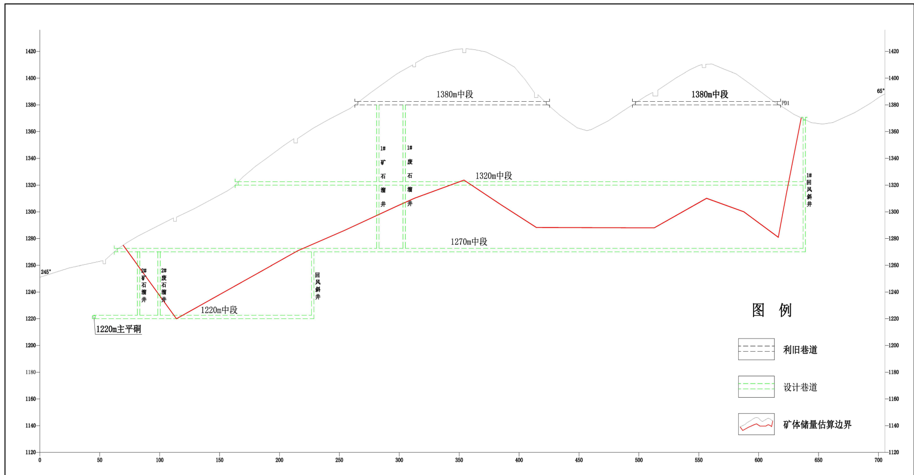
图 1-2 I 号矿体开拓系统纵投影图
