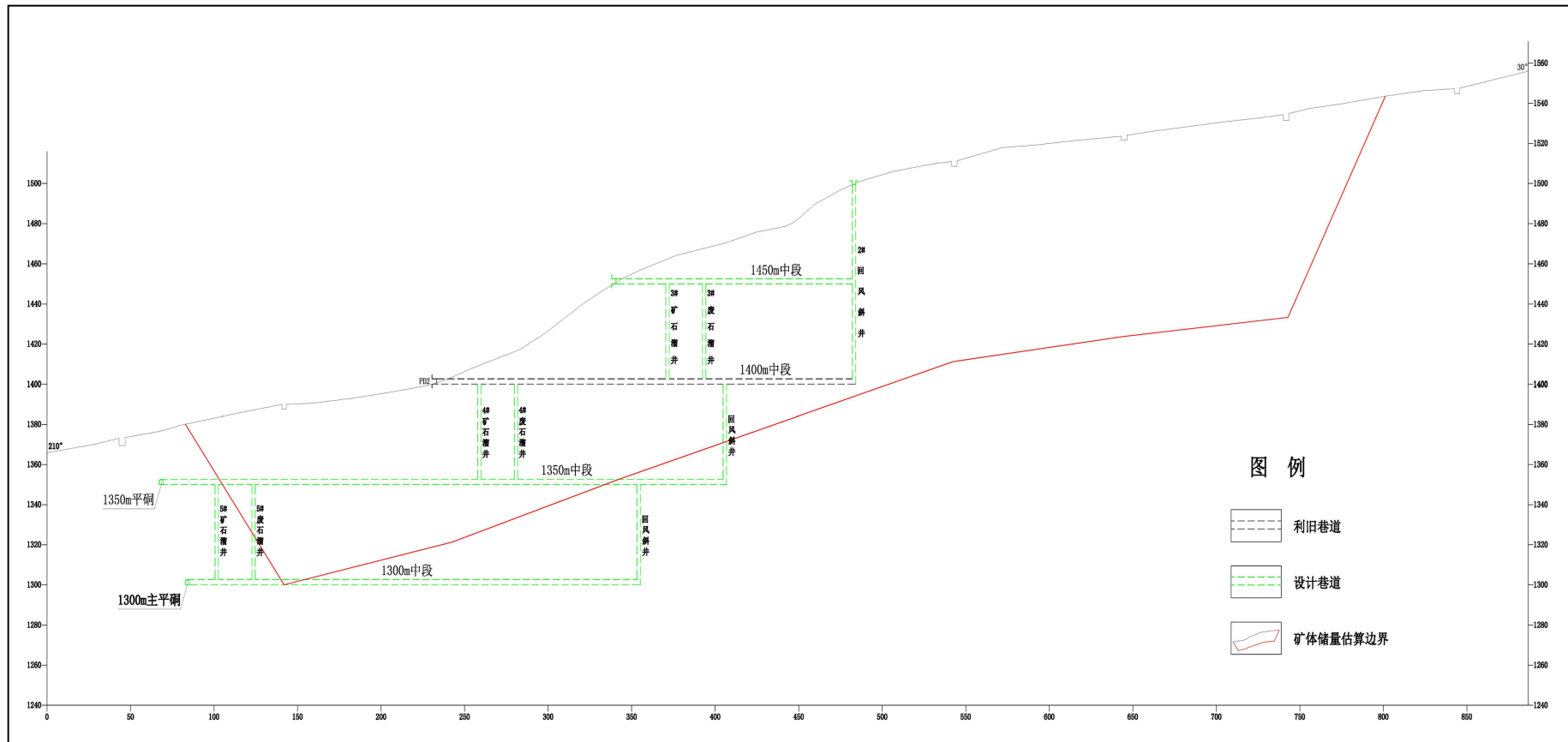
图 1-3 II 号矿体开拓系统纵投影图
