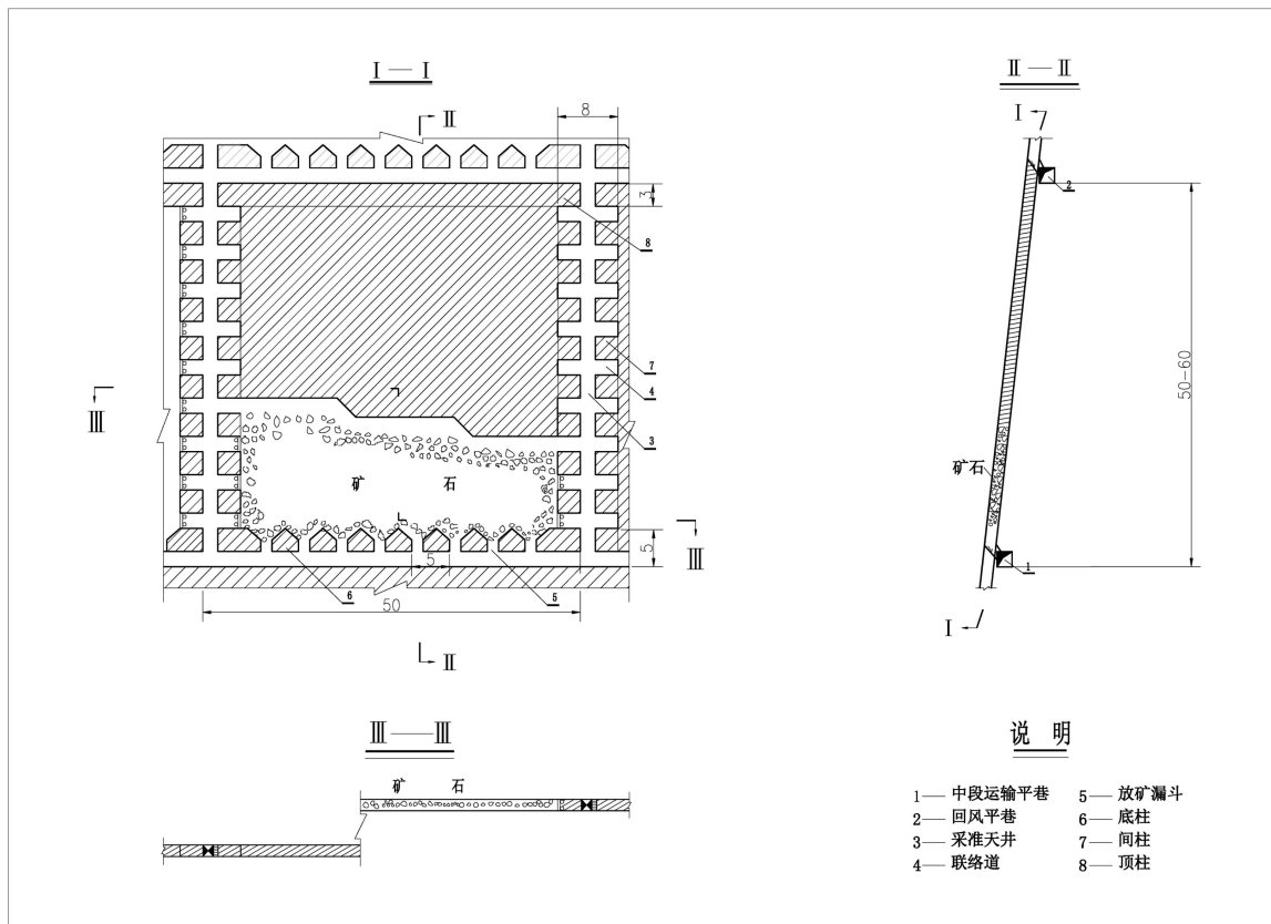
图 1-5 浅孔留矿法采矿方法图
