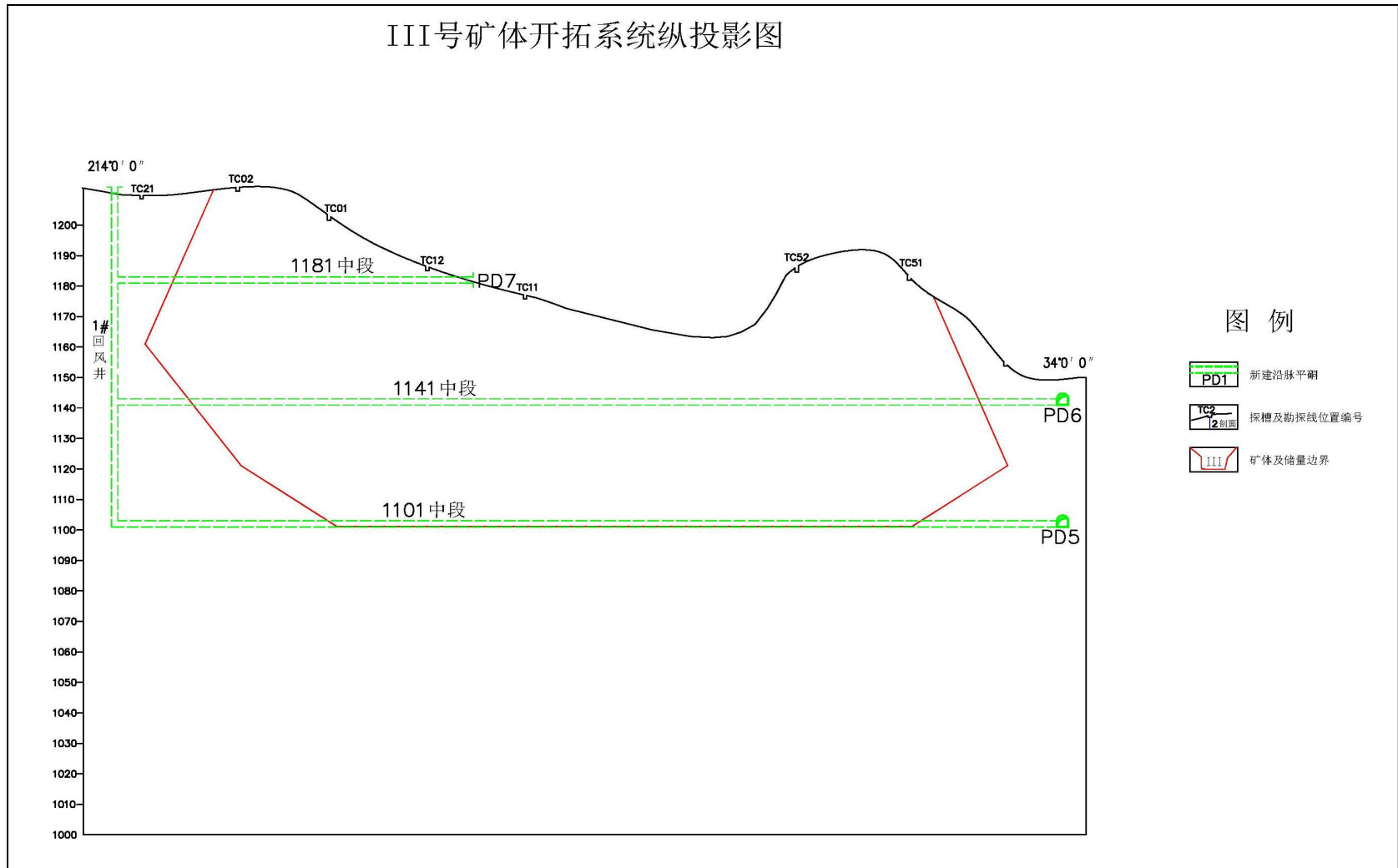
图 1-2 III号矿体开拓系统纵投影图
