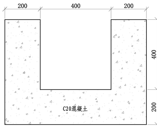
图 5-2 截排水沟断面图
