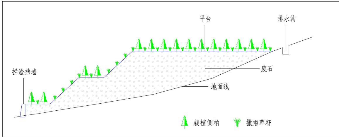
图 5-4 废石场植树典型设计图
