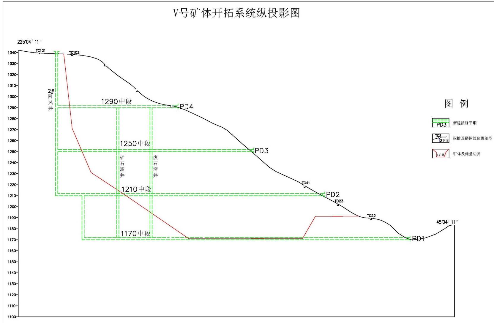
图 1-3 V号矿体开拓系统纵投影图
