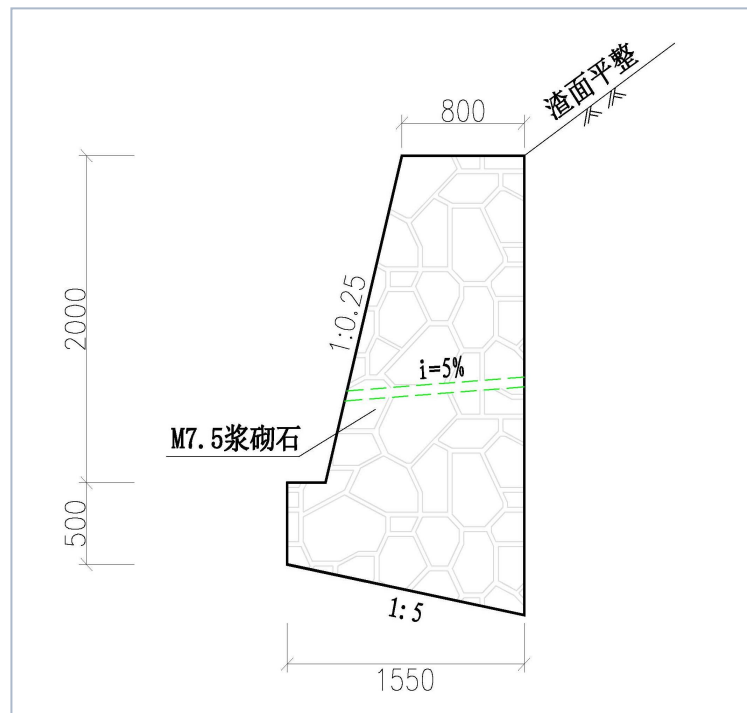
图 5-1 拦渣挡墙断面设计图
