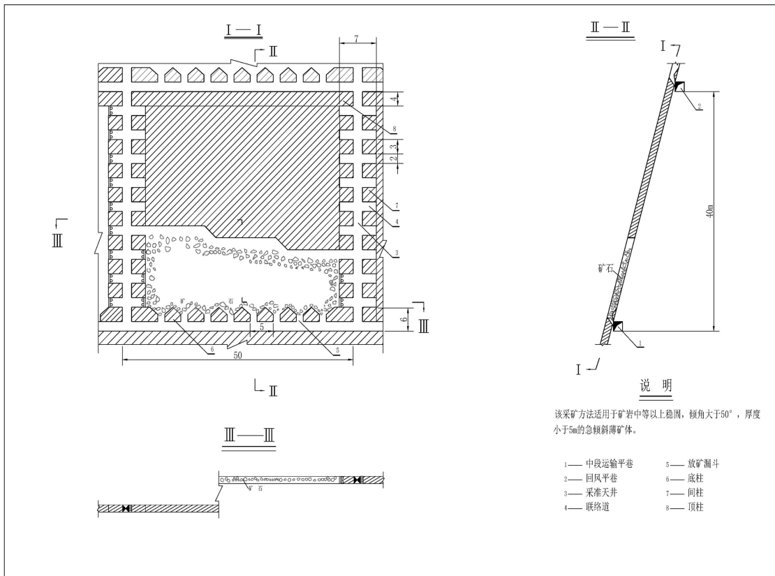
图 1-5 浅孔留矿法采矿方法图
