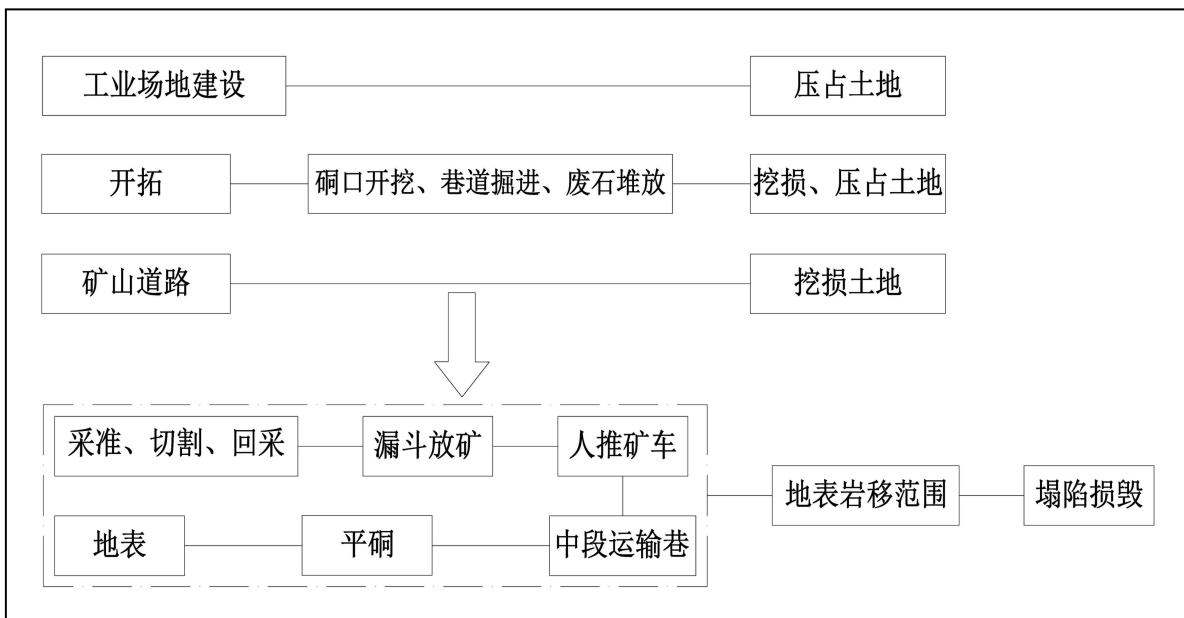
图 3-2 生产工艺流程与土地损毁环节分析图
