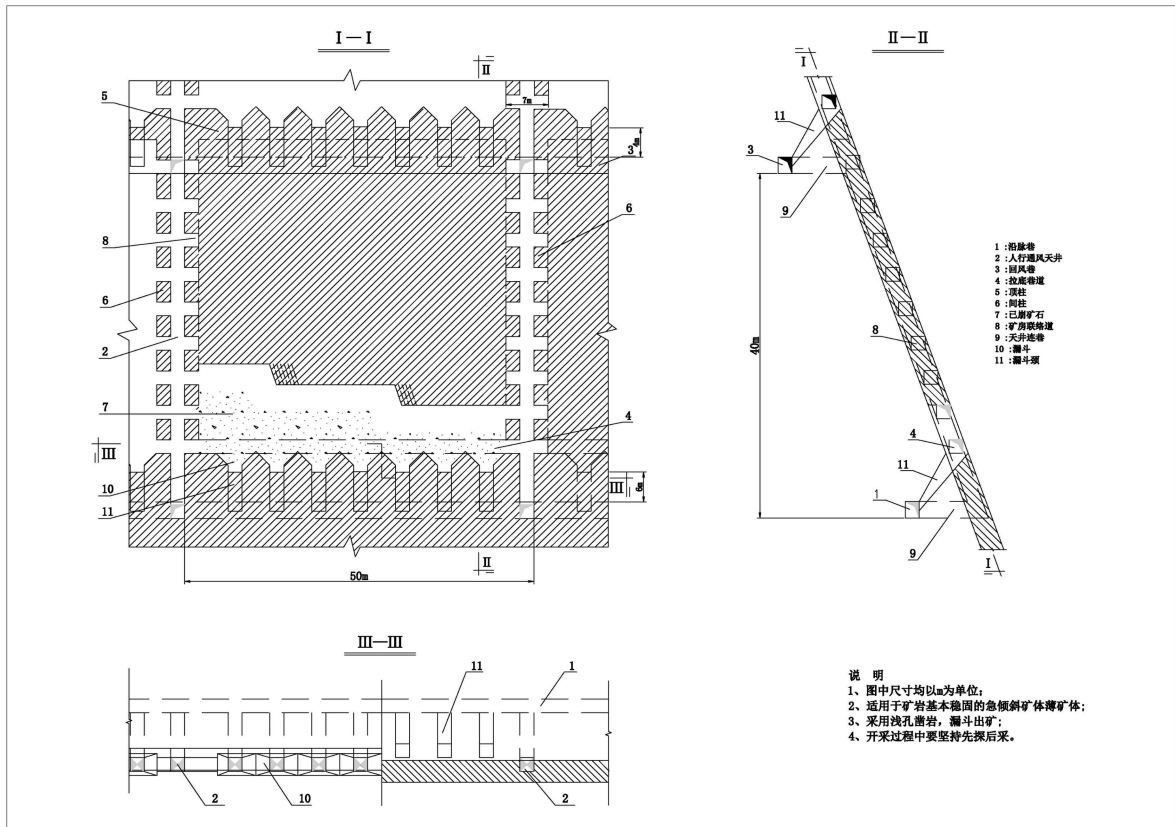
图 1-4 浅孔留矿法采矿方法图
