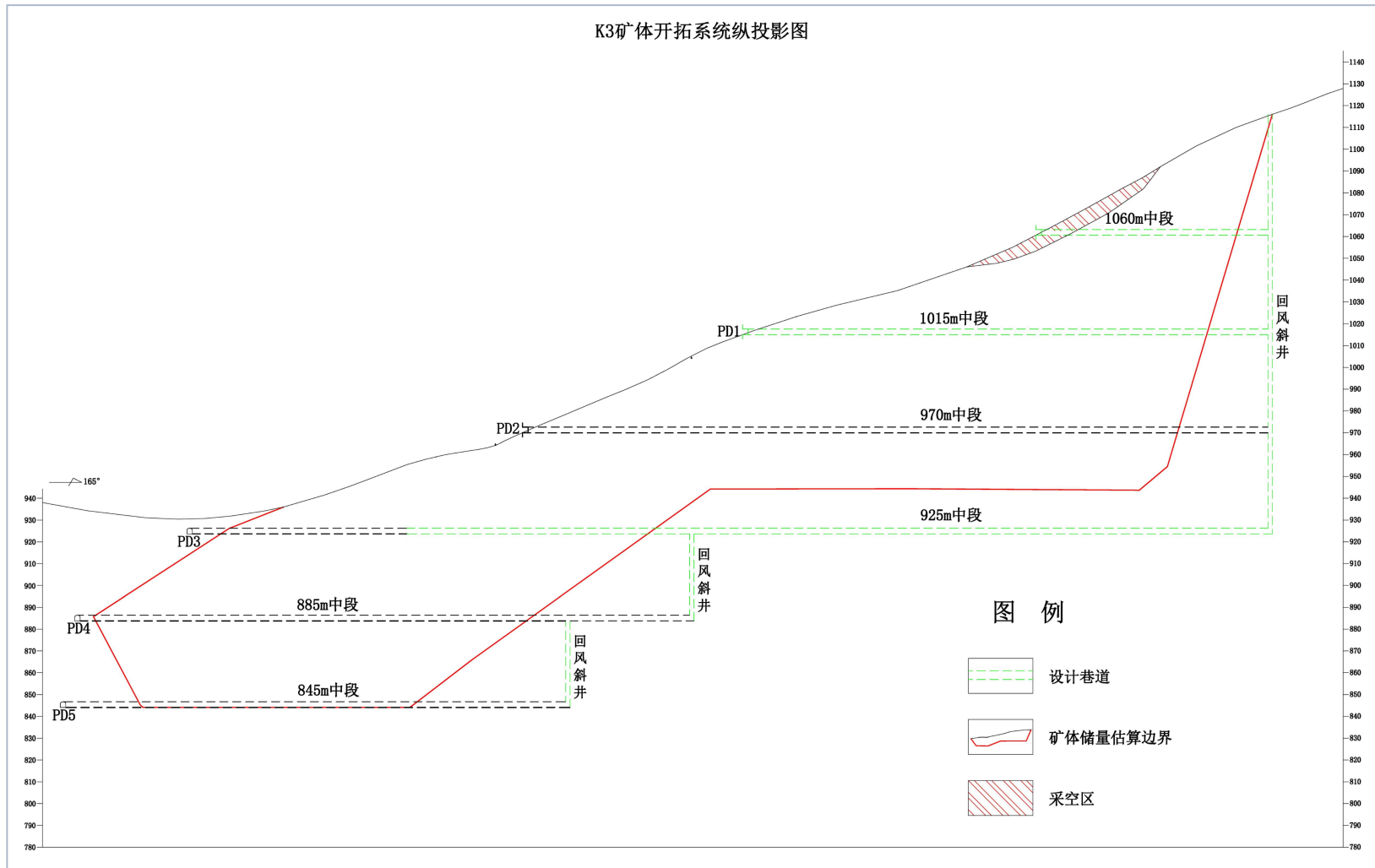
图 1-2 K3 矿体开拓系统纵投影图
