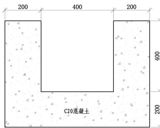
图 5-2 截排水沟断面图
