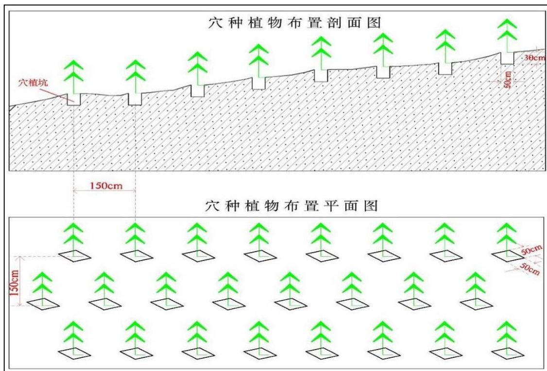
图 5-4 栽植乔木典型设计图
