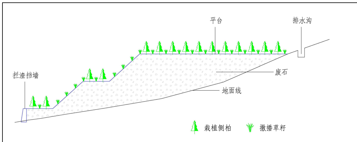
图 5-5 废石场植树典型设计图
