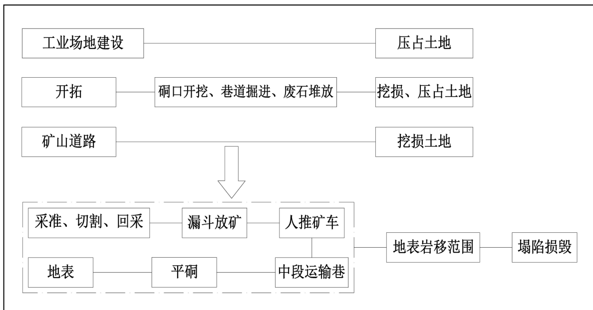
图 3-5 生产工艺流程与土地损毁方式分析图
