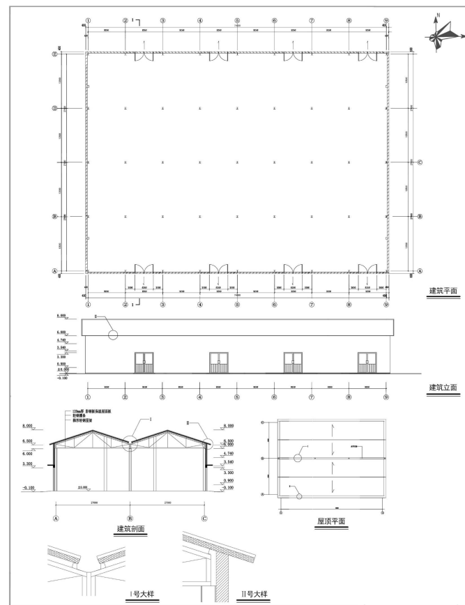
1号成品仓库设计图
