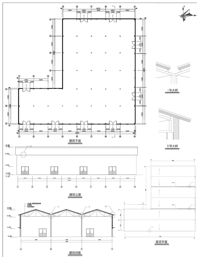
1号生产厂房设计图
